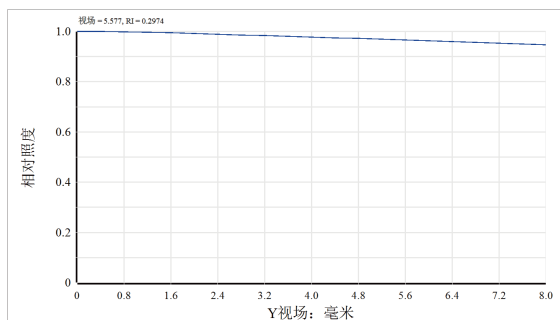
相对照度
