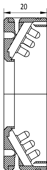
剖视图 A-A
