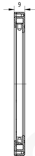
剖视图A-A
