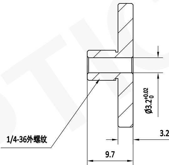
剖面E-E
